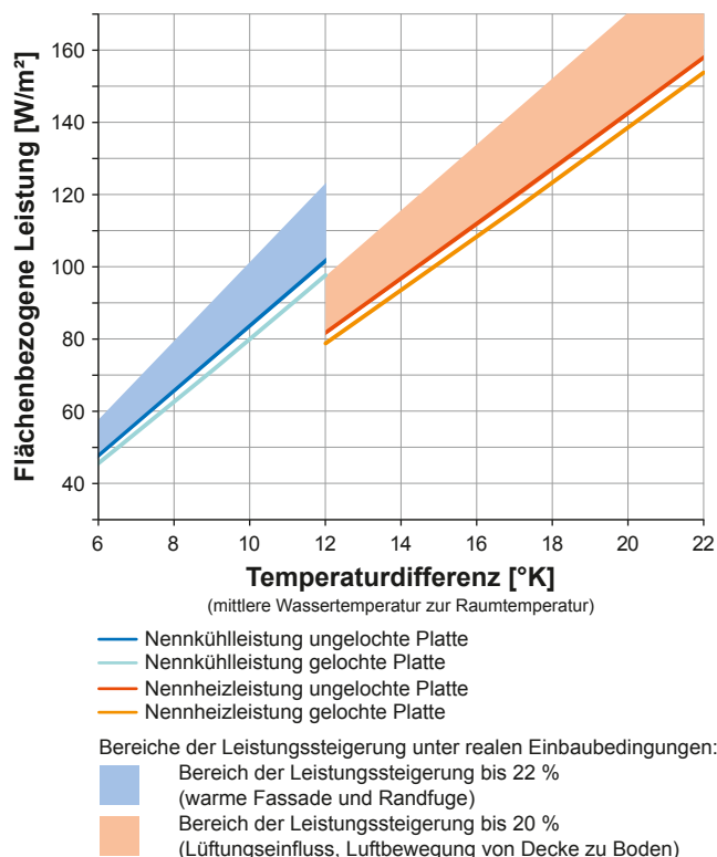
Heiz-/Kühlleistung Uponor ThermoTop M, geprüft nach DIN EN 14240 bzw. DIN EN 14037
