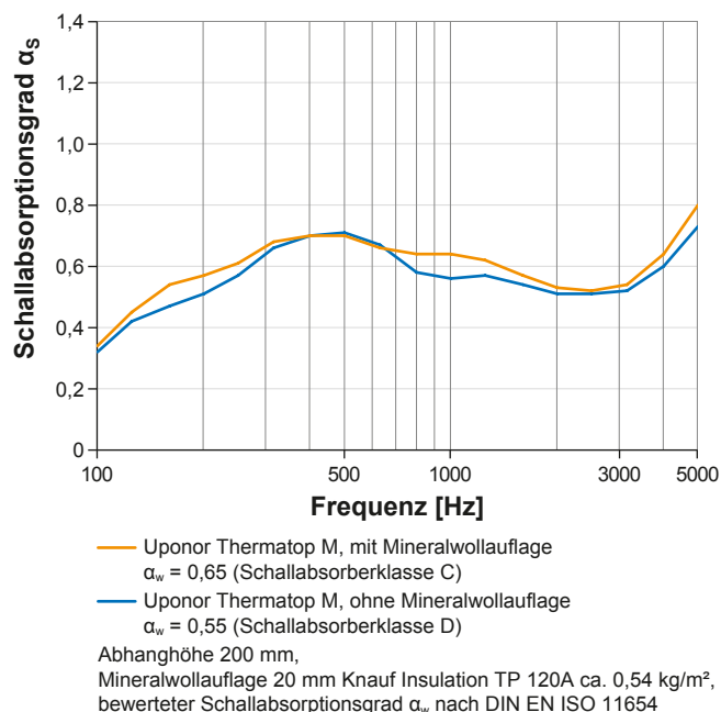
Schallabsorption Uponor ThermoTop M, geprüft nach DIN EN ISO 354
